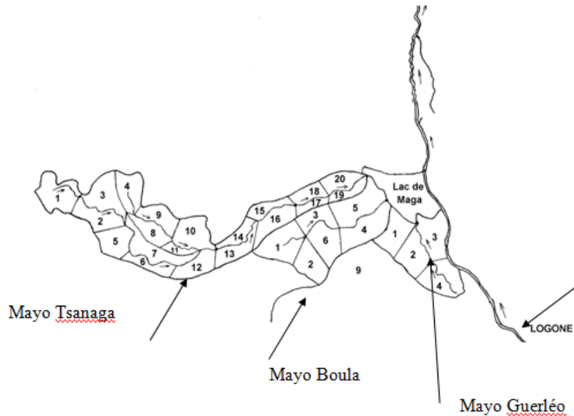
Figure 32. Schéma du système fluvial du lac Maga et les bassins et sous-bassins versant correspondants.
