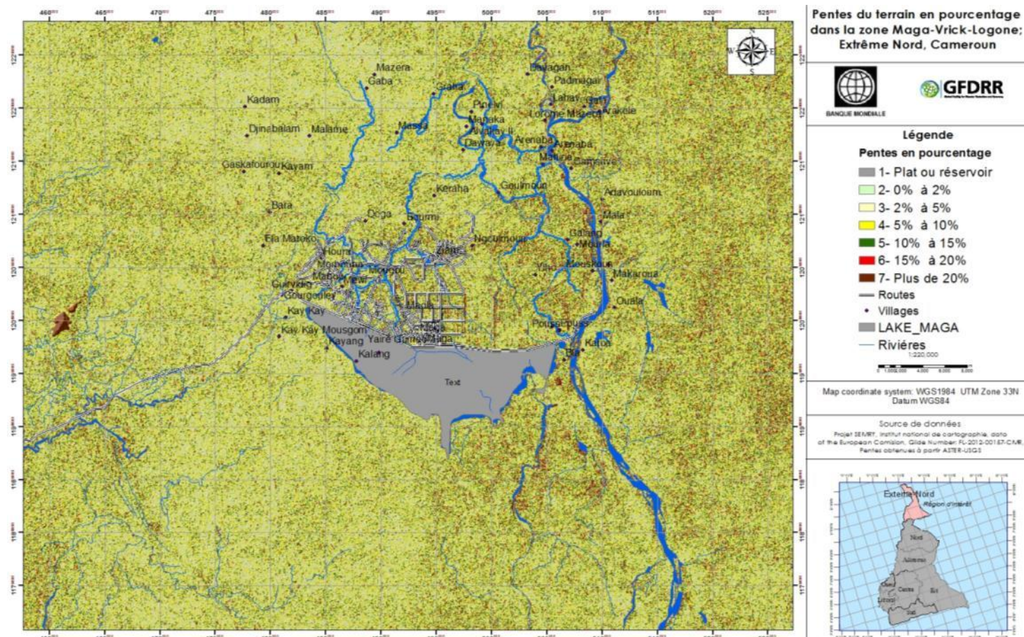
Figure 25. Pentes en pourcentage dans la zone du barrage de Maga.
