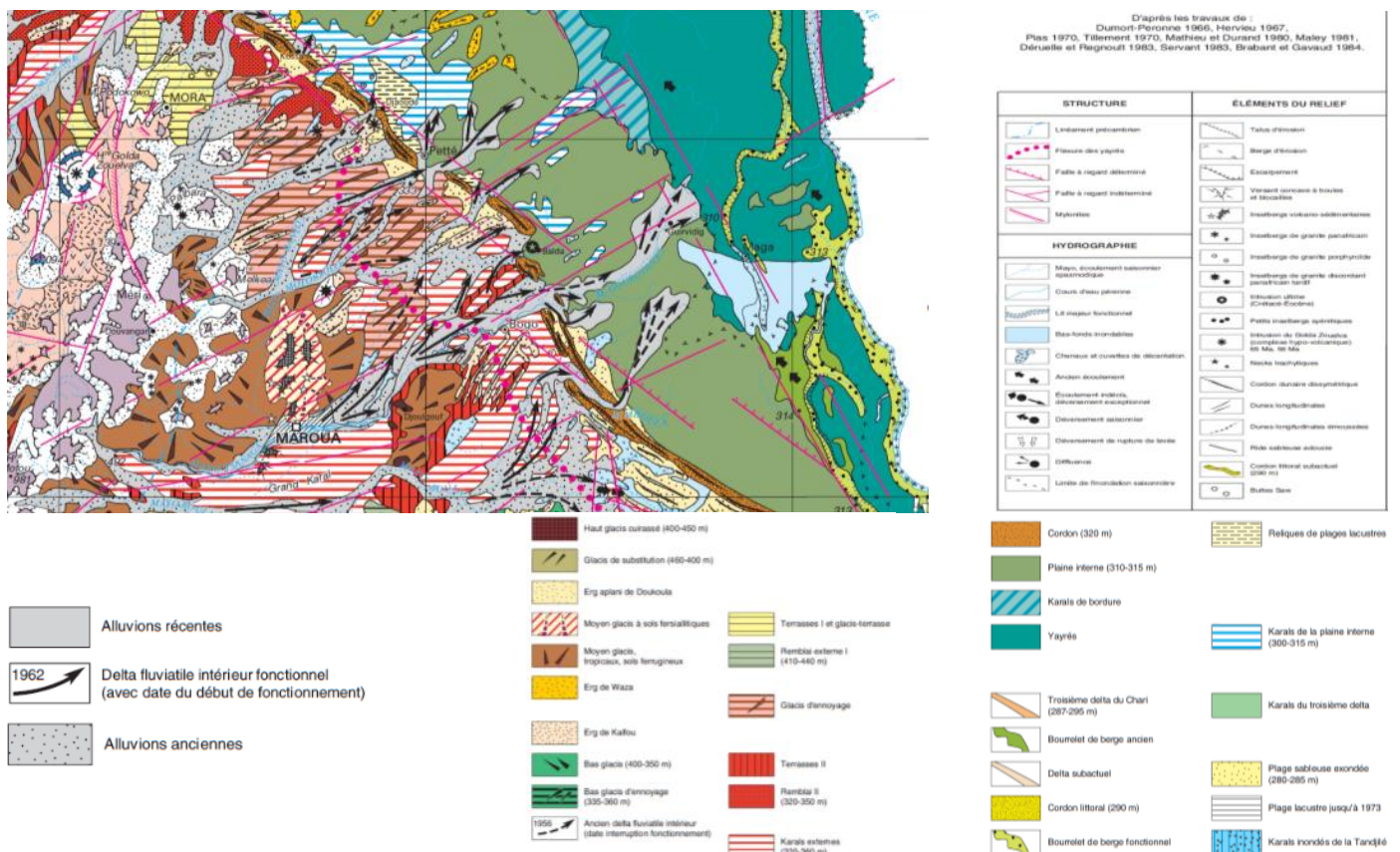
Figure 45. Carte géomorphologique des environs de Maga et Maroua (Seignobos, Iyébi-Mandjek et al. 2000)
